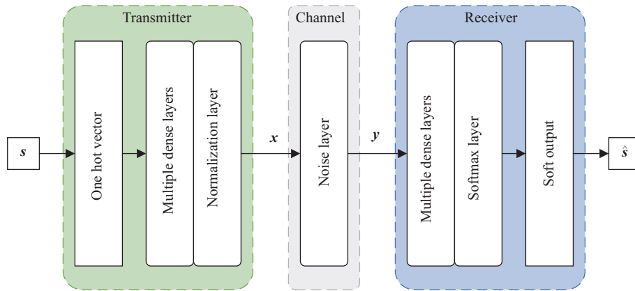
图 8 (网络版彩图) 用自编码器构建端到端通信模型的简单结构 [37]
