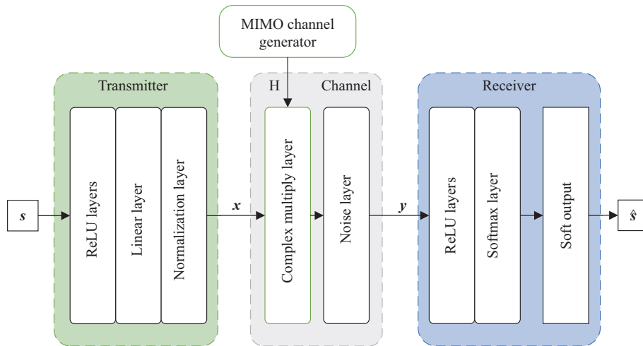
图 9 (网络版彩图) 用自编码器构建的 MIMO 端到端通信模型结构 [37]
