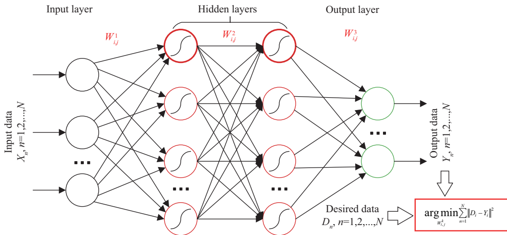
图 1 (网络版彩图) 监督学习示例: 多层神经网络学习
