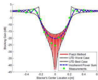
图 3 毫米波传播障碍物阻挡实验 (原图来源 网络)
