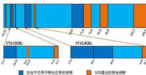
图 1 毫米波通信主要频段
