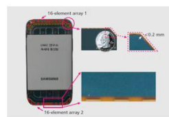
(a) 个人移动终端毫米波阵列天线
